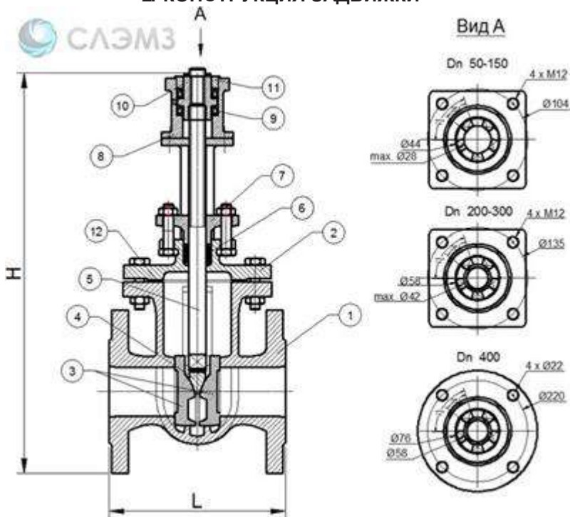
Рис.1 Конструкция задвижки
